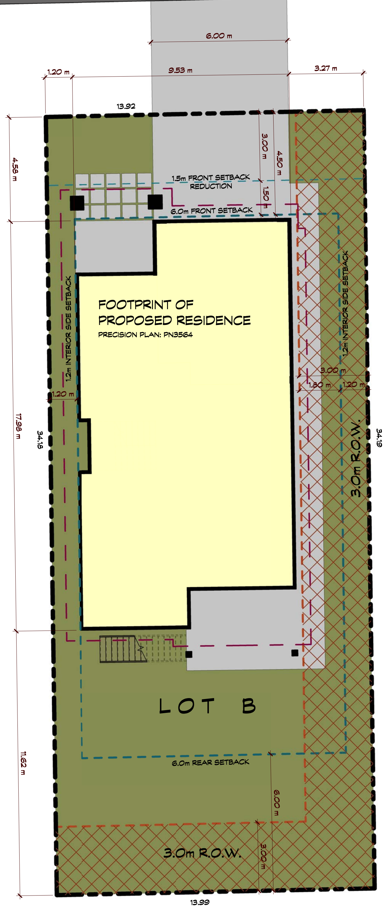
SITE PLAN 1:100
